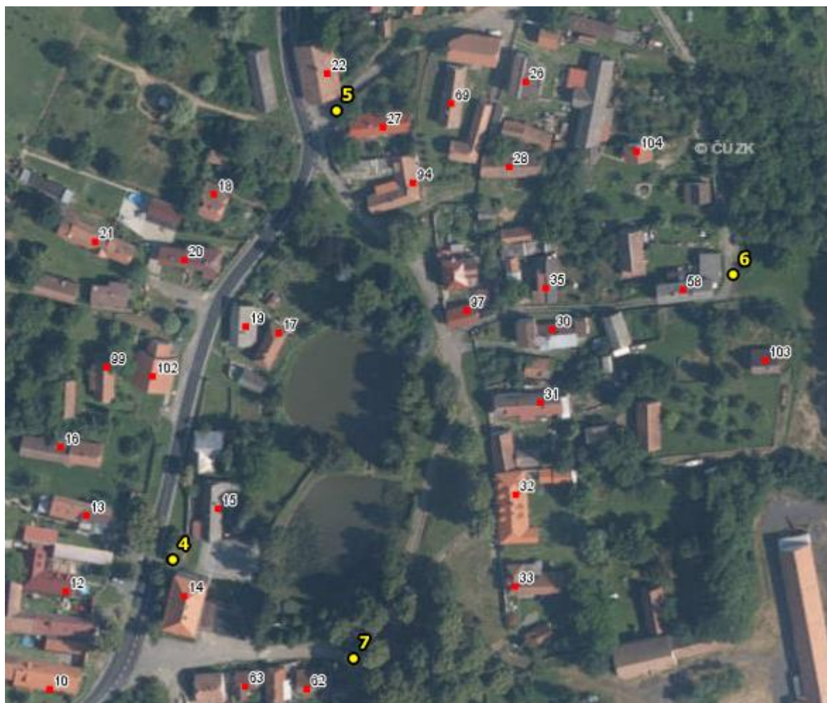
Umístění hlásičů v obci Hraběšín – detail 2
